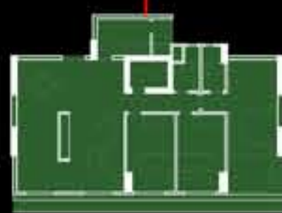
TYPE F5, 3 BEDROOMS GFA : 115sqm
